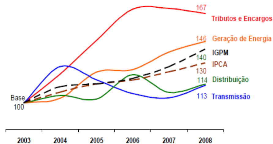
Evolução do Custo dos Componentes da Tarifa de Eletricidade vs. Índices de Inflação Base 100 = 2003
